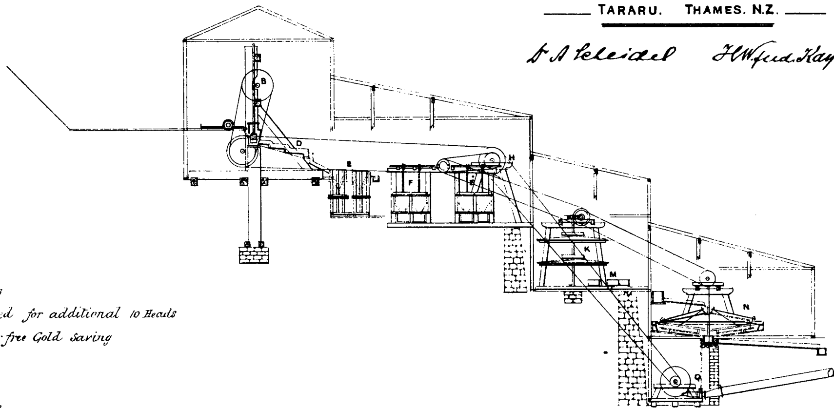
LONGITUDINAL SECTION
