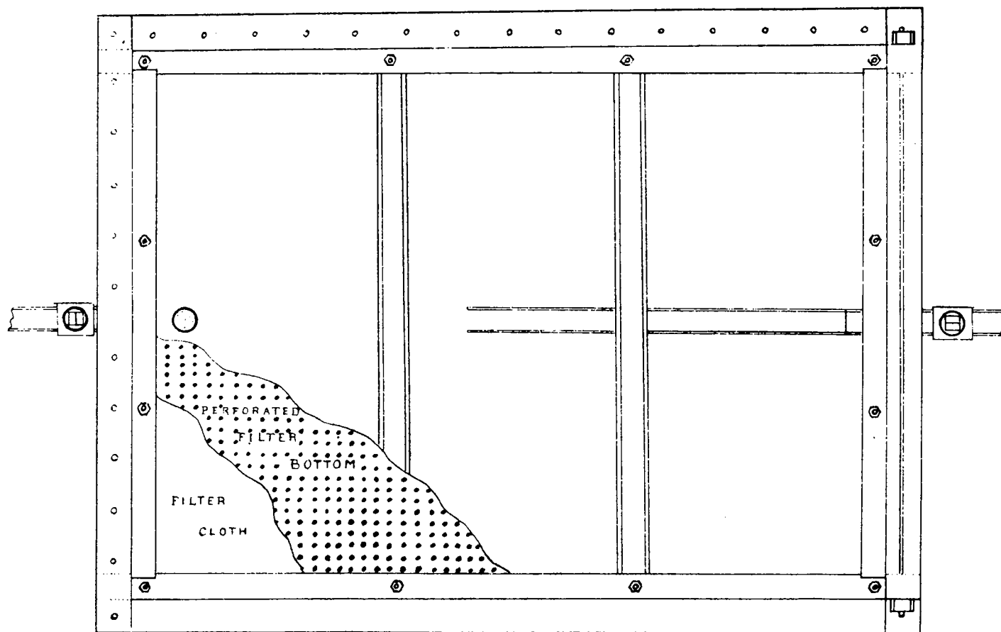
— HORIZONTAL SECTION —
