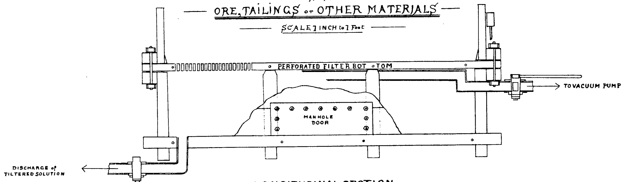
— LONGITUDINAL SECTION —
